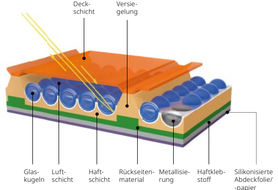
Aufbau mit eingekapselten Glaskugeln
