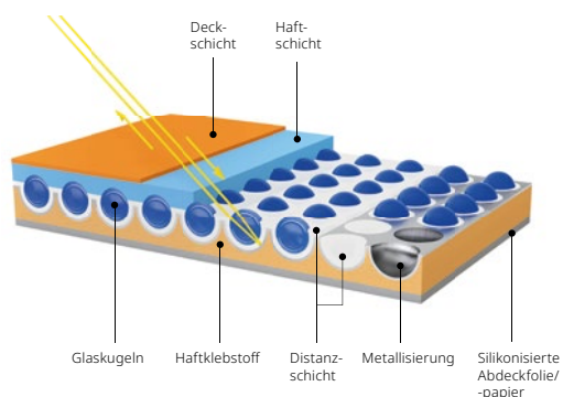
Aufbau mit eingebetteten Glaskugeln
